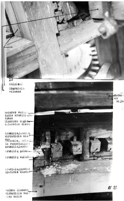
Malūno kepurės fragmentai iš vidaus. Aut. nuotr. 1981 m.
