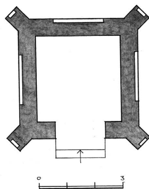
8 brėž. Pilviškių varpinės planas. Sudarė A. Rupeika
