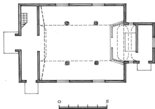
33 brėž. Parausių koplyčios planas. Sudarė A. Rupeika
