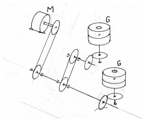
V. Federavičiaus motorinio malūno planas
