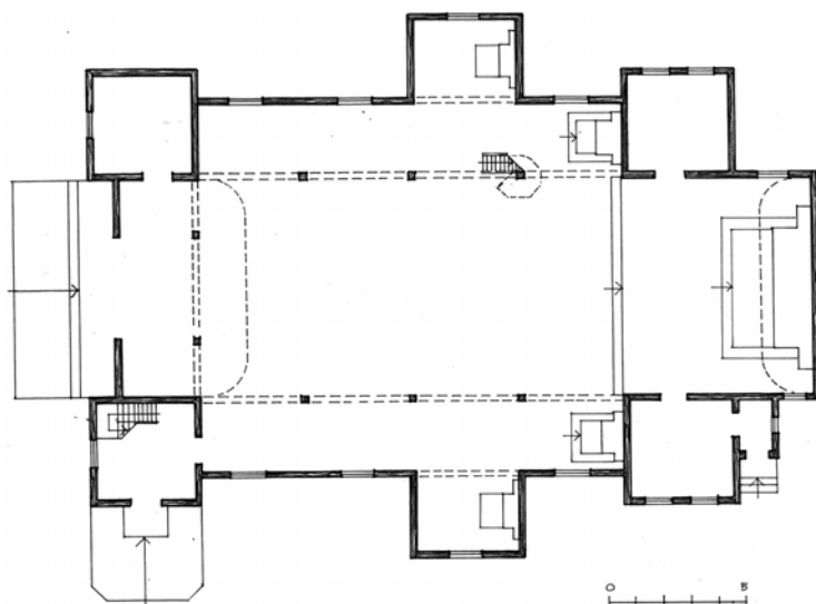
25 brėž. Bagotosios bažnyčios plano schema. Sudarė A. Rupeika
