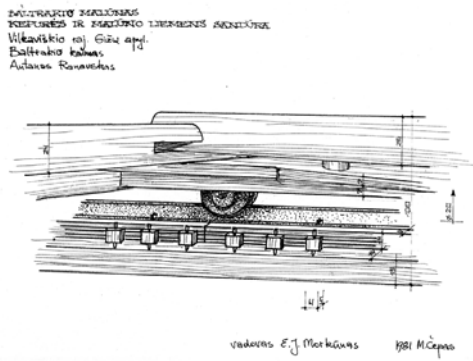
Malūno kepurės ir malūno liemens sandūra. Braižė M. Čepas, 1981 m.
