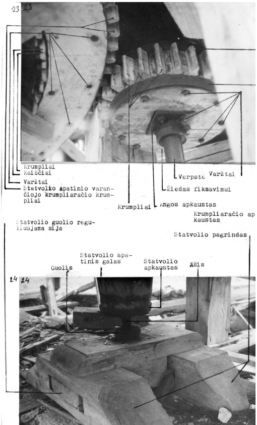
Malūno vidaus mazgai. Aut. nuotr. 1981 m.
