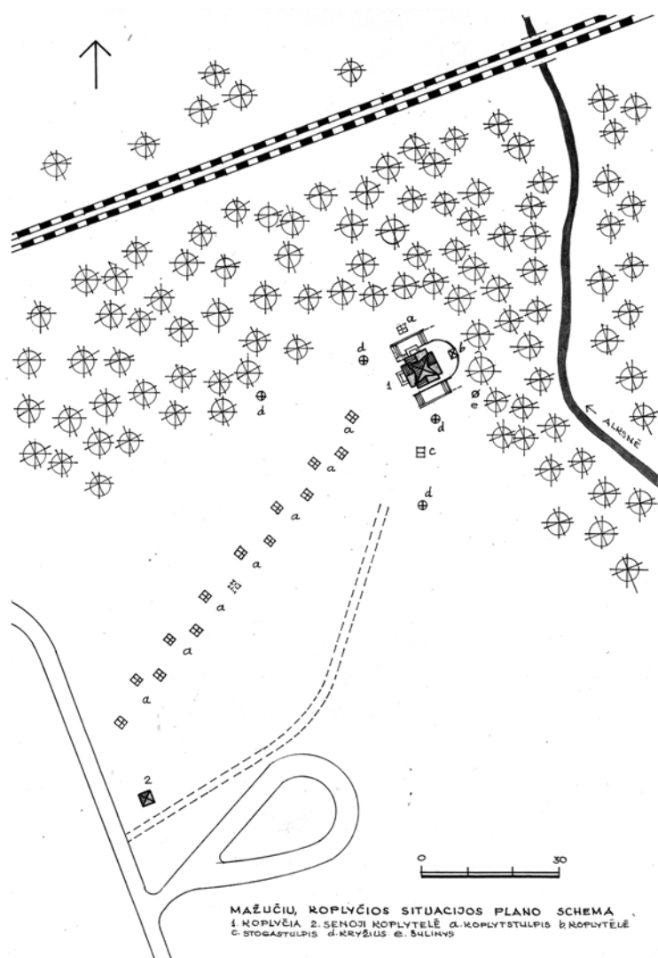
29 brėž. Mažučių kopyčios statinių komplekso situacijos plano schema. Sudarė A. Rupeika
