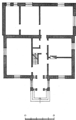
9 brėž. Pilviškių klebonijos planas. Sudarė A. Rupeika
