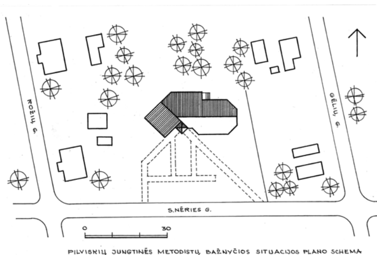
11 brėž. Pilviškių jungtinės metodistų bažnyčios situacijos plano schema. Sudarė A. Rupeika
