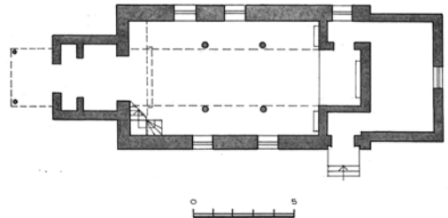
35 brėž. Žaliosios bažnyčios planas. Sudarė A. Rupeika
