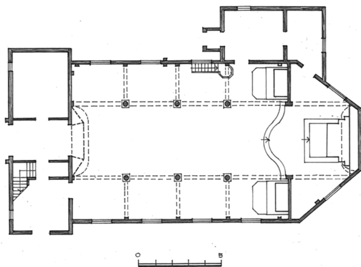
18 brėž. Alksnėnų bažnyčios planas. Sudarė A. Rupeika
