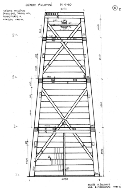
Vinkšnupių vėjo malūno sienos išklotinė.
