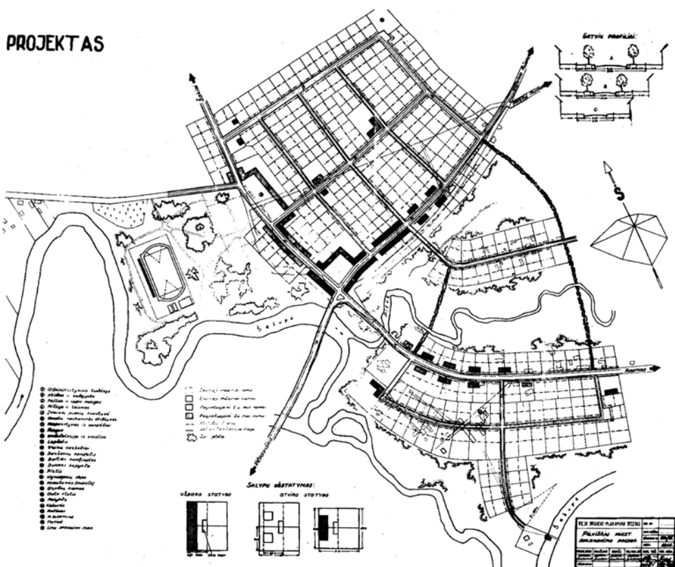
9 pav. 1945 m. miestelio atstatymo projektas
