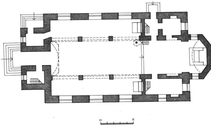
27 brėž. Didvyžių bažnyčios planas. Sudarė A. Rupeika
