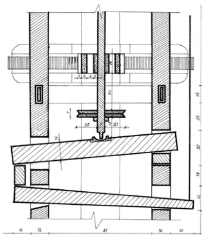
Timinciškių malūno girnų stovas.
