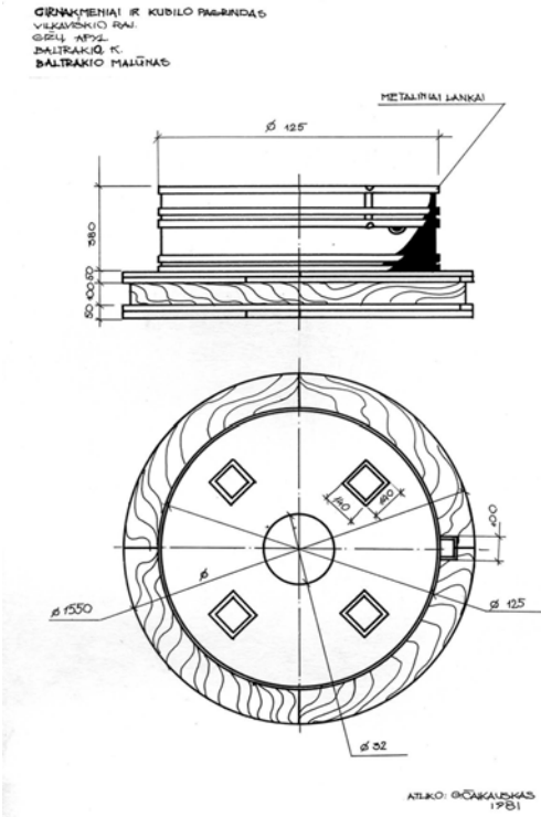
Girakmeniai ir kubilo pagrindas. Braižė Gintaras Čaikauskas. 1981 m.
