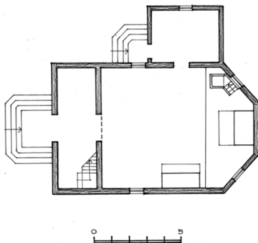
31 brėž. Paežerių kapinių koplyčios planas. Sudarė A. Rupeika
