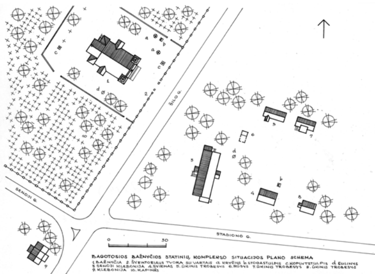
24 brėž. Bagotosios bažnyčios statinių komplekso situacijos plano schema. Sudarė A. Rupeika
