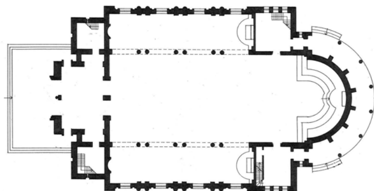
7 brėž. Pilviškių katalikų bažnyčios planas. Sudarė A. Rupeika
