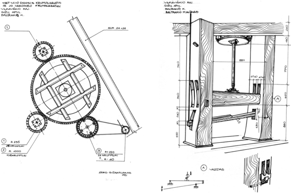
Statvolio didysis krumpliaratis ir jo varomieji krumpliaraičiai. Braižė G. Čaikauskas. 1981 m.
