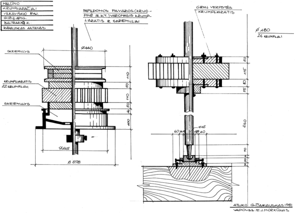
Papildomos pavaros (kruopinė ir kt.) varomasis krumpliaratis ir skriemuliai. Girnų verpstės krumpliaratis. Braižė G. Čaikauskas. 1981 m.
