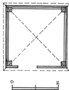
19 brėž. Alksnėnų varpinės planas. Sudarė A. Rupeika
