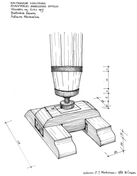
Statvolio apatinis guolis. Braižė Mindaugas Čepas. 1981 m.
