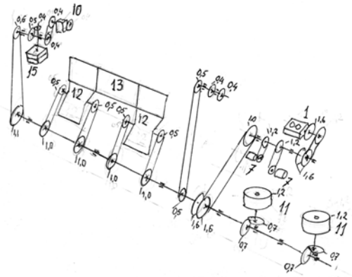
A. Kromienės motorinio malūno kinematinė schema. Sukamų įrenginių numeriai atitinka brėžinio eksplikacijos numerius: 1 – variklis „Laval“, 7 – elektros generatorius, 10 – kaušinis gabentuvas, 11 – gornos, 12 – valcai, 15 – plokščiasietis. Skriemulių ir krumpliaraičių skersmenys pažymėti metrais
