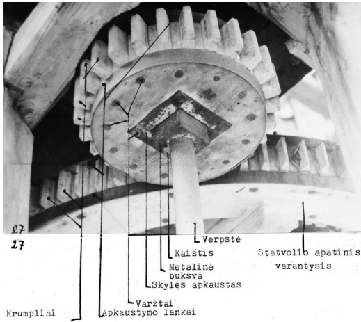
Malūno statvolio apatinio krumpliaračio ir girnų verpstės fragmentai. Aut. nuotr. 1981 m.
