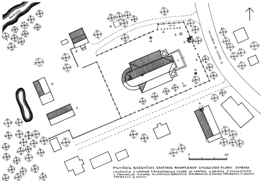
5 brėž. Pilviškių bažnyčios statinių komplekso situacijos plano schema. Sudarė A. Rupeika
