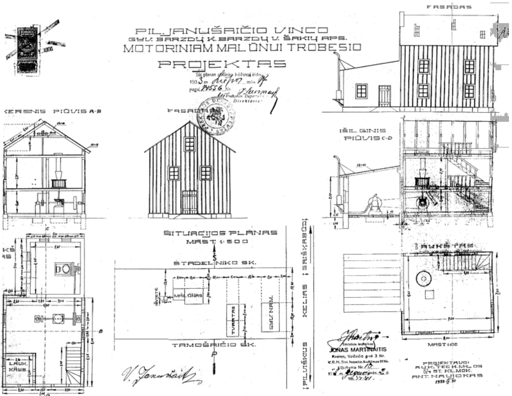
V. Janušaičio motorinio malūno planas
