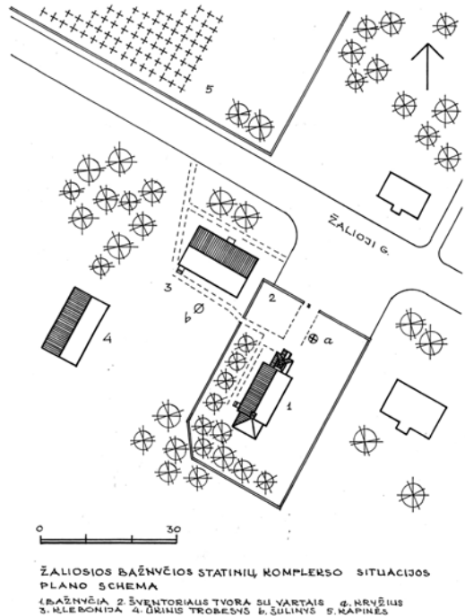
34 brėž. Žaliosios bažnyčios statinių komplekso situacijos plano schema. Sudarė A. Rupeika
