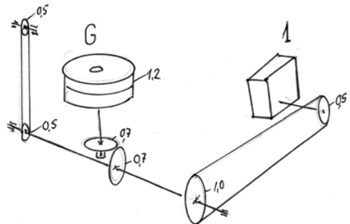
V. Janušaičio motorinio malūno kinematinė schema: 1 – motoras, G – girnos. Skriemulių, krumpliaracių ir girnų skersmenys pažymėti metrais
