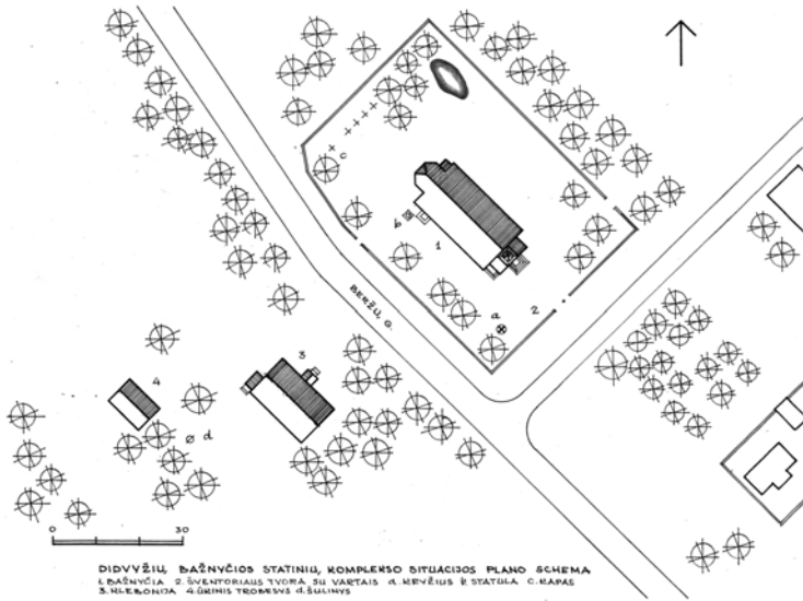
26 brėž. Didvyžių bažnyčios statinių komplekso situacijos plano schema. Sudarė A. Rupeika
